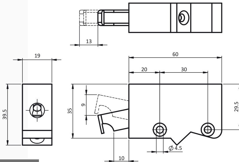
Šteljući nosač kuhinjskog elementa, univerzalni
